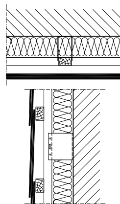
Konsola aluminiowa profil U z pionowym łączeniem podstawowym i poziomym nośnym
