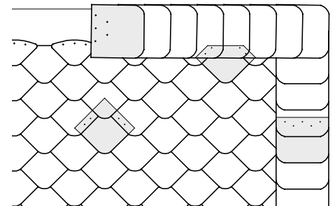
Zakończenie górne i boczne z nałożonym rzędem zamykającym
