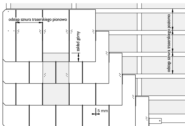
Przykład: Format 30 x 60 cm, z rogami prostokątnymi
