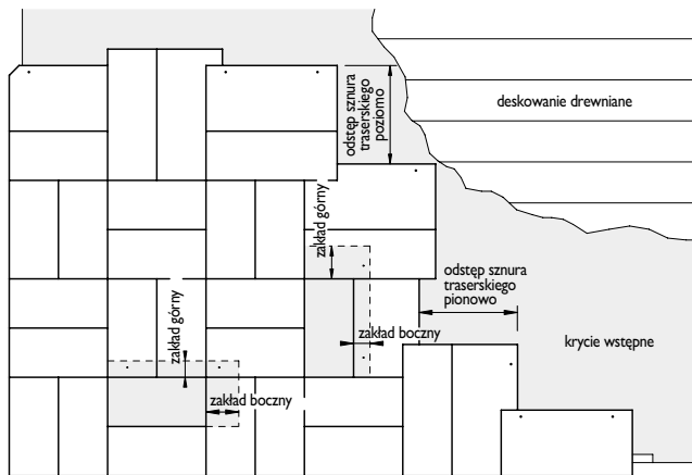
Krycie mozaikowe lewe, 40 x 20 cm, z docinaniem krawędziami szczytowymi
