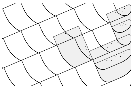
Wykończenie deski szczytowej w sposób podwójny
