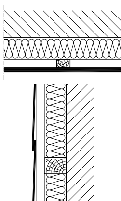
Pionowe łączenie nośne na poziomym łączeniu podstawowym
