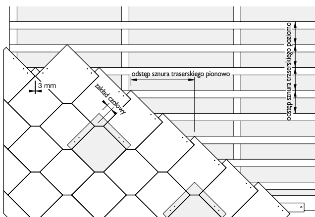
Przykład: Format 30 x 30 cm, ze ściętymi rogami, z docinanym kryciem szczytu
